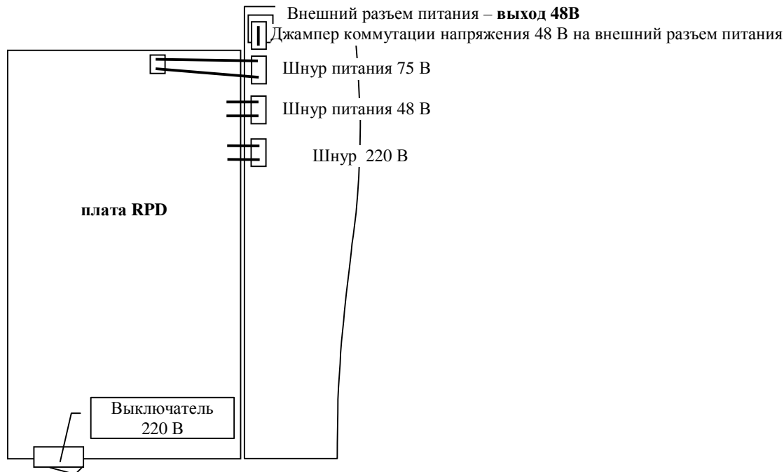
Рис. 46. Схема расположения узлов модем-мультиплексора MC04-DSL.F-xxx-220V.
